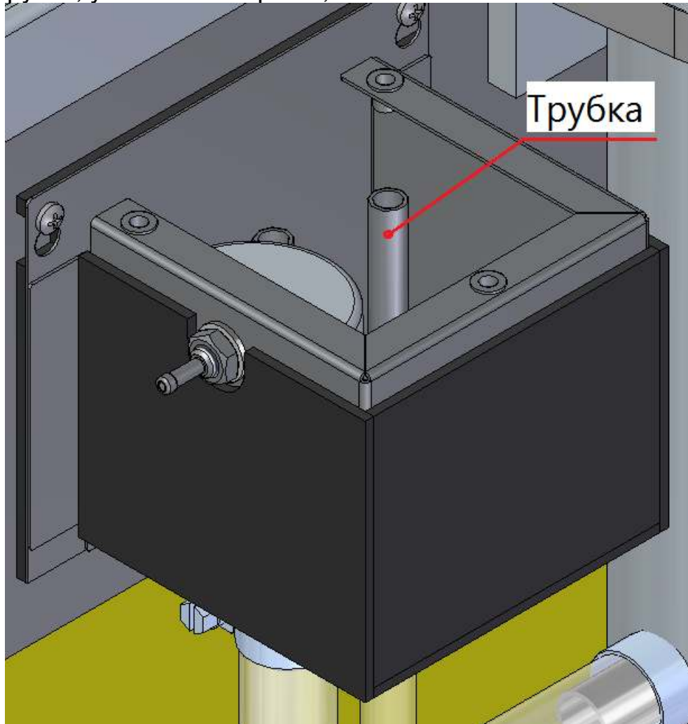
Рис. 5 Расположение трубки
